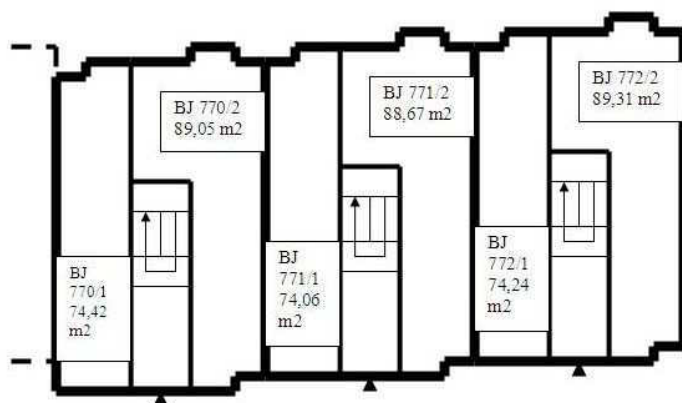
1. nadzemní podlaží
