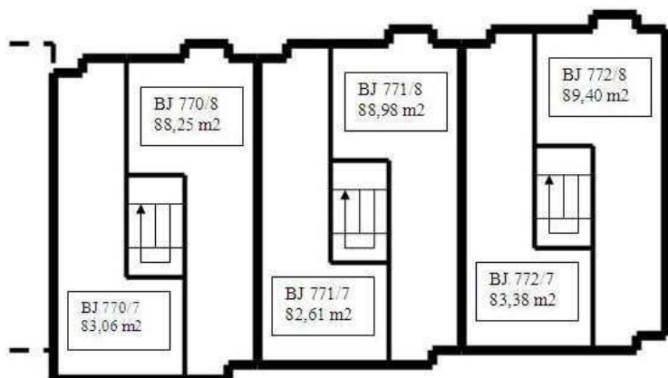
4. nadzemní podlaží
