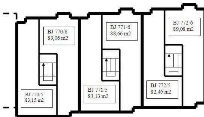
3. nadzemní podlaží
